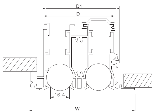
KVSLS3800 FRAME -SN-
