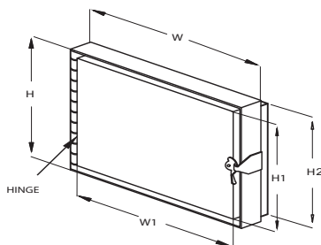
MODEL K60 (HAD) HINGED, FLUSH DOOR
